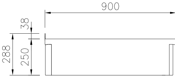
Zij aanzicht
